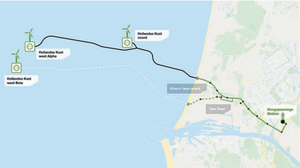
Het tracé van de elektriciteitskabels op zee en land voor het aansluiten van de drie toekomstige windparken voor de kust van Noord-Holland. Afbeelding: TenneT
