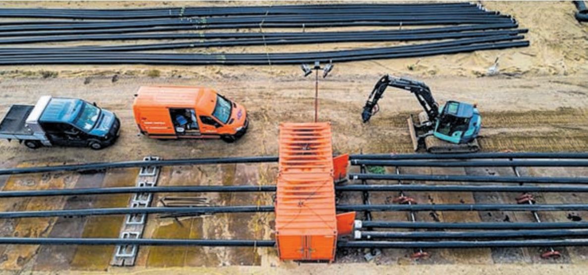
In de oranje container worden de mantelbuizen aan elkaar gelast. Foto: aangeleverd
