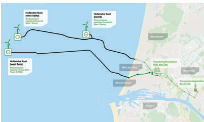
Op deze kaart is te zien waar zich de windparken West Alpha, West Bèta en Noord zich bevinden en hoe ze zijn aangesloten. Afbeelding: TenneT
