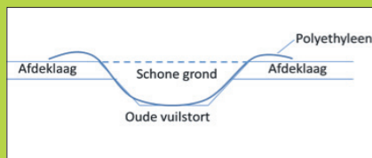
Stap 3: Aanbrengen polyethyleen folie + schone grond
