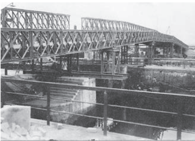
Tijdelijke Bailey-brug over de Kleine en de Zuidersluis, Noordzeekanaalsluizen IJmuiden
