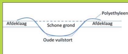
Stap 3: Aanbrengen polyethyleen folie + schone grond
