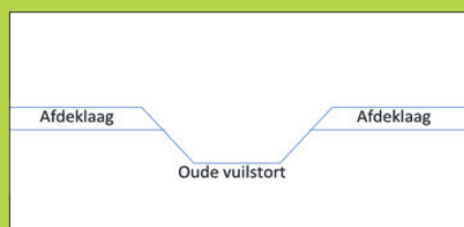
Stap 2: Ontgraven kabel- en leidingtracé
